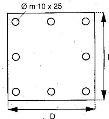
Burner mounting flanges Befestigungsflansch des Brenners
