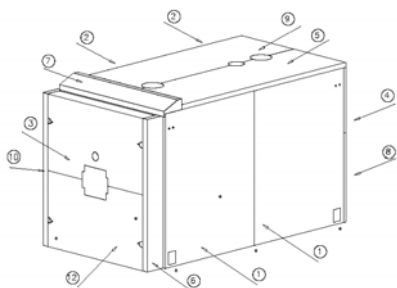
Jacket Ummantelun
